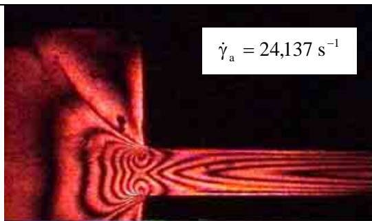
Figure-6- Cliché de biréfringence induite par l'écoulement du PEbd-IUPAC à 150°C
